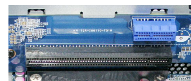
Zwei PCI-Express Slots: X16 und X1
